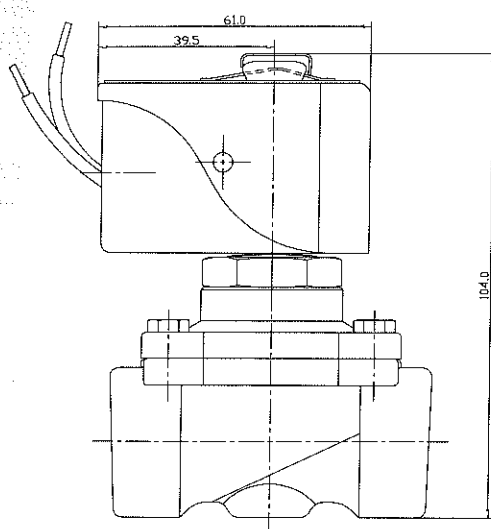
Desenho 1 - Válvula N.F. NPT/BSP
