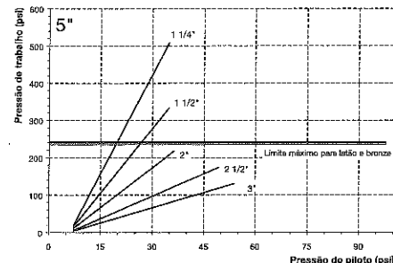
Diâmetro do atuador - 125 mm
