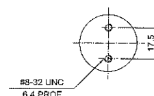
Vista de A
